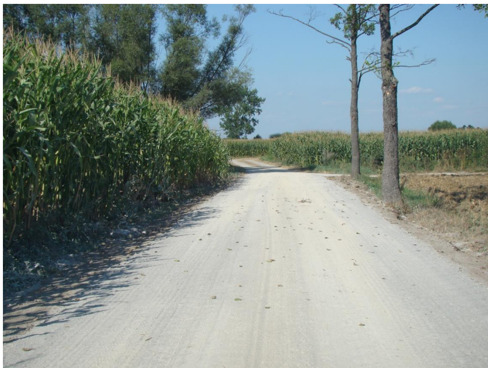
Fot. Nr 5a – Widok w km 0+925 po wykonaniu - koniec modernizacji odcinka drogi. Data wykonania: stan w dniu 14 sierpnia 2020 r.
